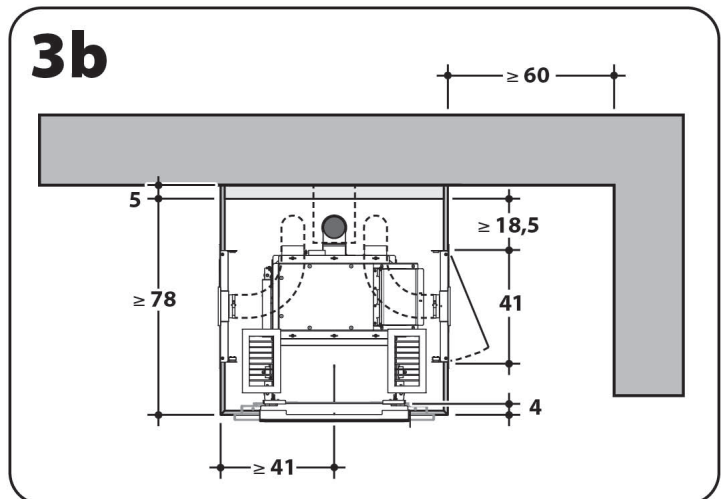
Exemple sur INSIDE S avec chargement à droite
