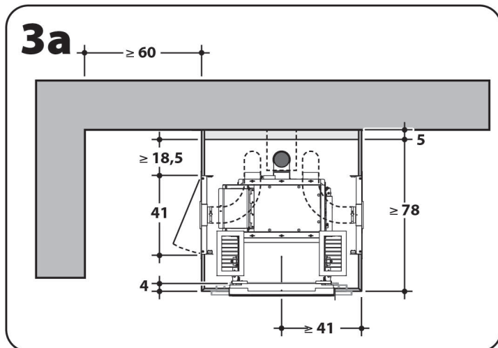
Exemple sur INSIDE S avec chargement à gauche
